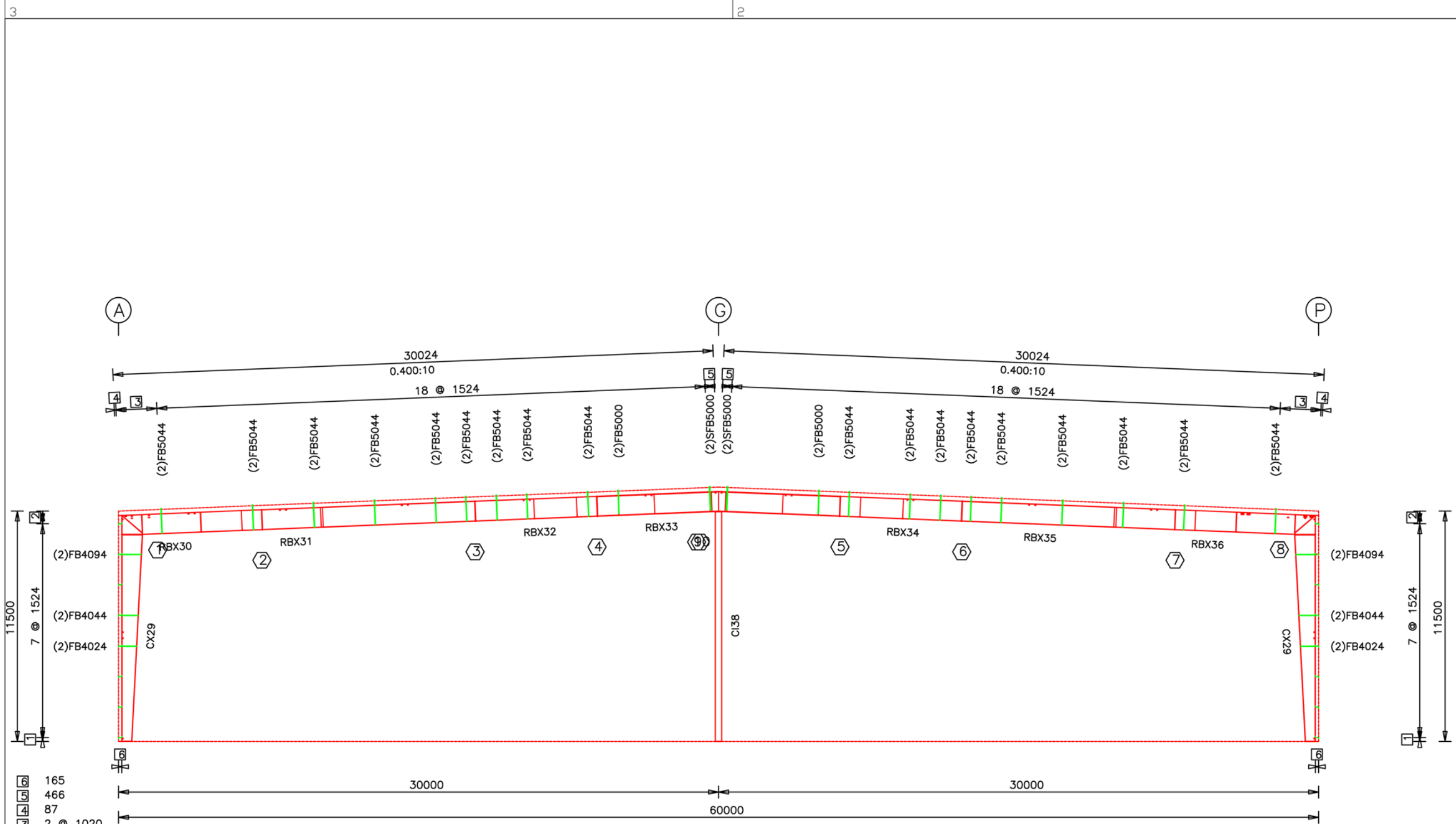
PORTICO TIPICO
