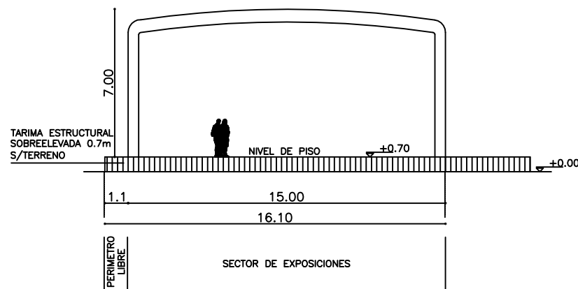
CORTE TRANSVERSAL
