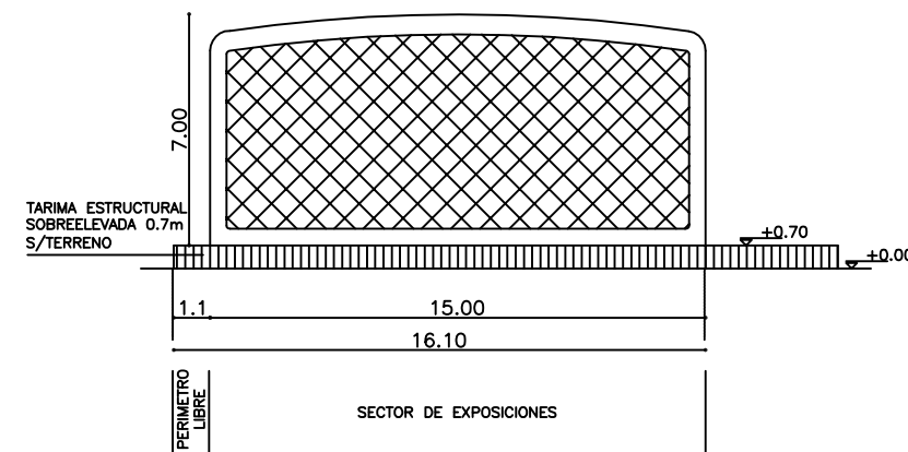
VISTA LATERAL
